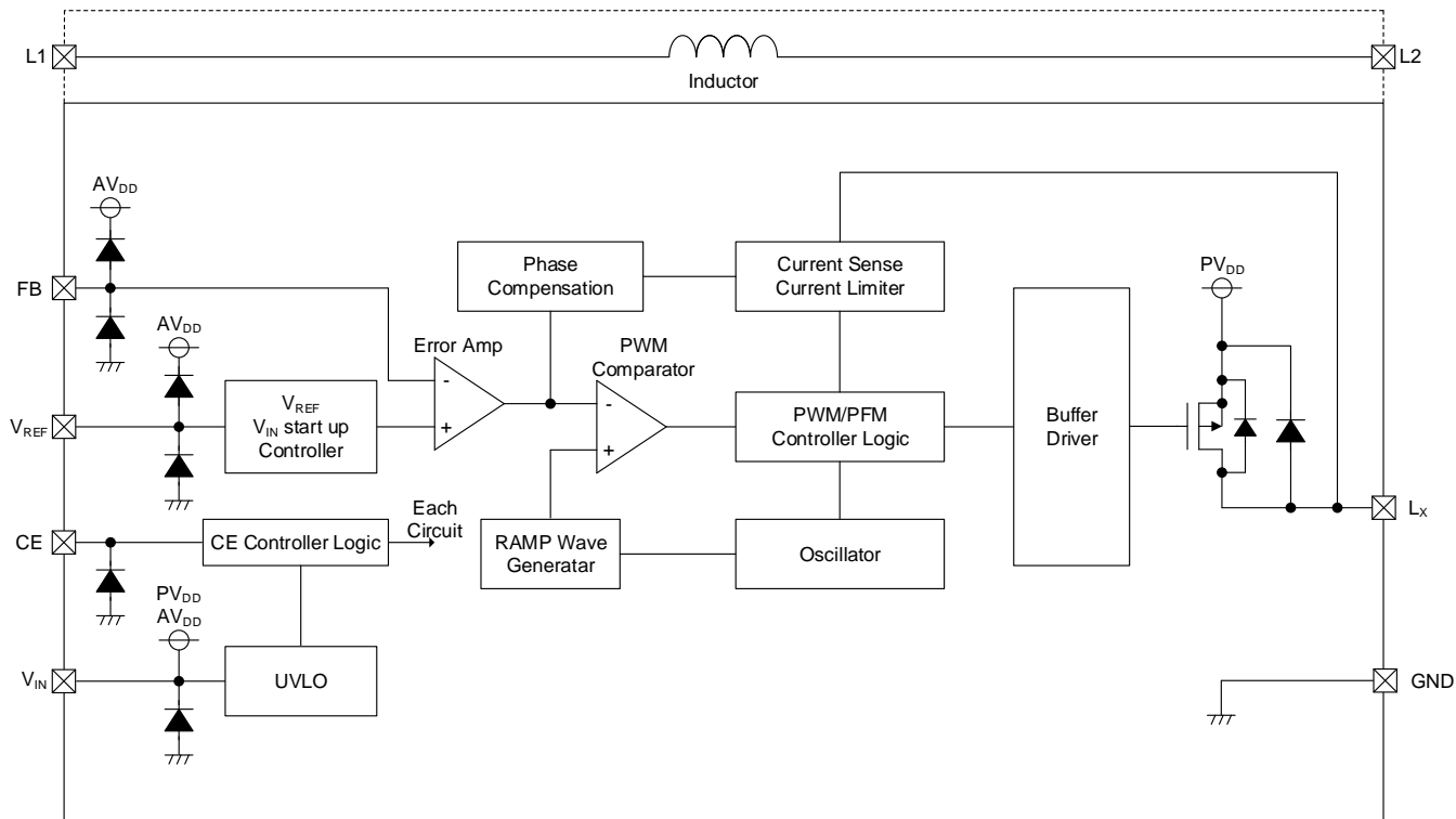
XCL303/XCL304 シリーズ ブロック図
