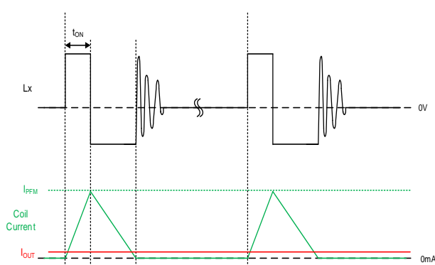
XCL303シリーズ：軽負荷時、動作例
