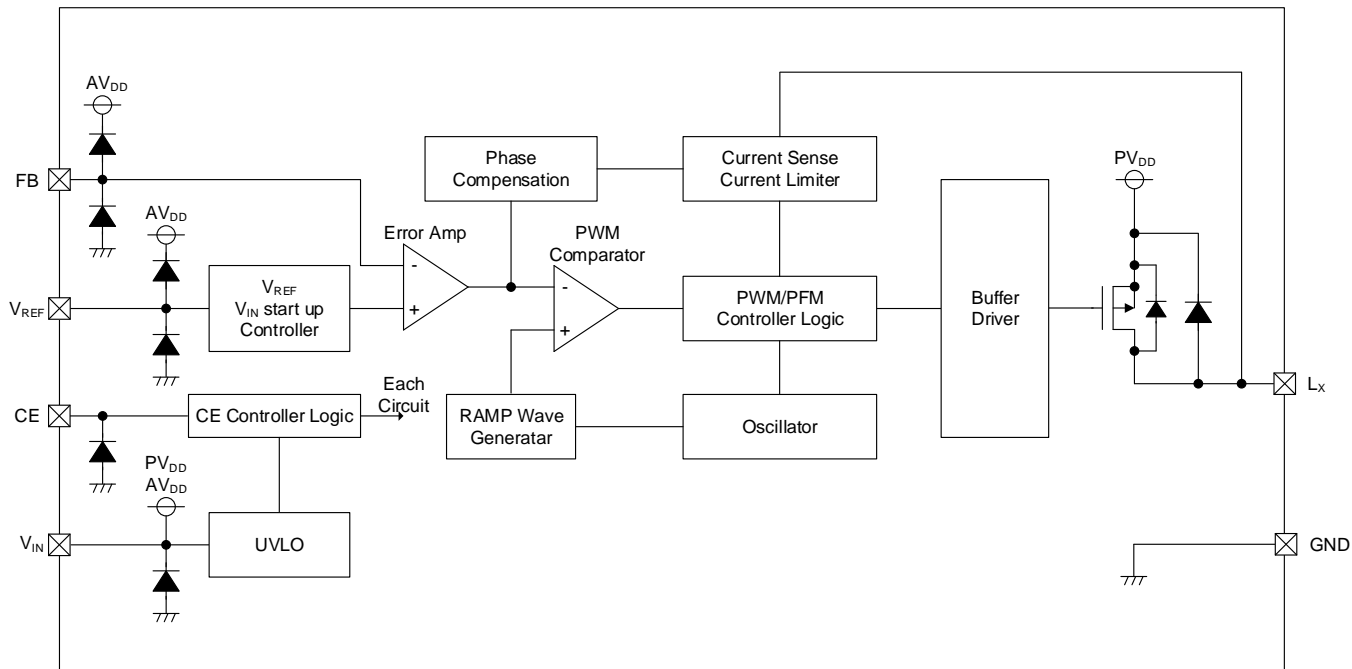
XC9307/XC9308 シリーズ ブロック図
