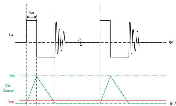
XC9307シリーズ：軽負荷時、動作例
